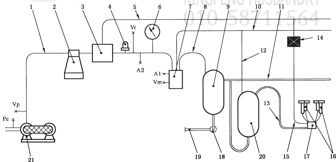
图2 管道式挤奶机示例
