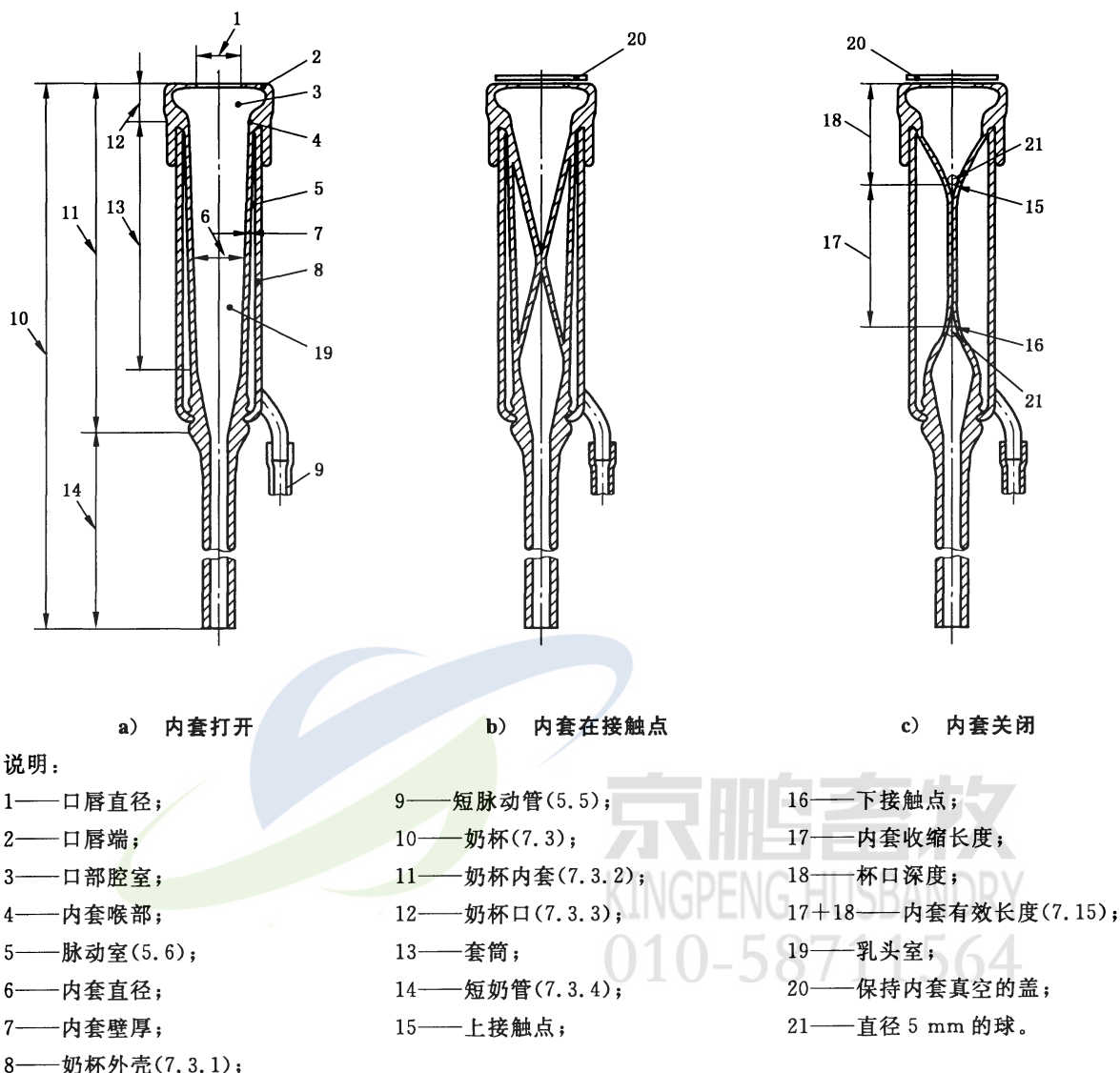
图 7 奶杯组成部件
